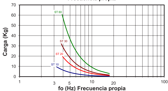
Frecuencia propia
