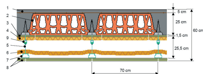
Forjado empleado para el ensayo
