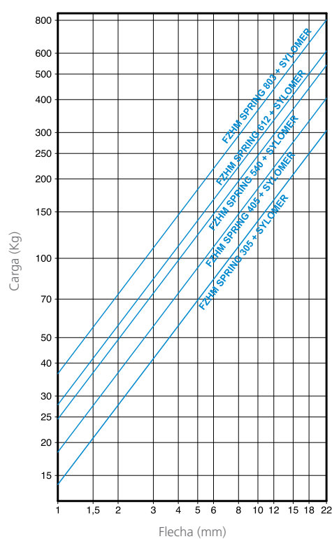
CURVAS DE CARGA - FLECHA FZHM SPRINGS + SYLOMER ®
