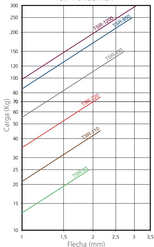
CARGA FLECHA ESTÁTICO TSR + SYLOMER ®
