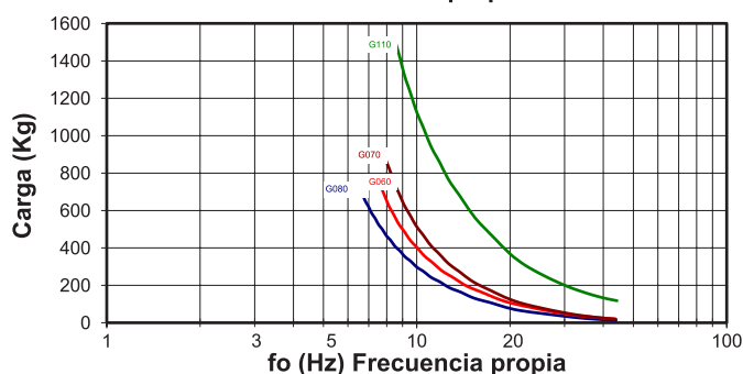
Frecuencia propia
