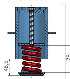
SECCIÓN A-A POSICIÓN A CARGA MÁXIMA
