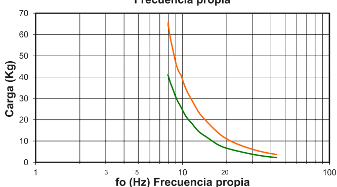
Frecuencia propia
