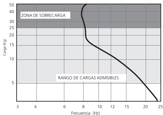
CURVA DE FRECUENCIA NATURAL EP Akustik + Sylomer
