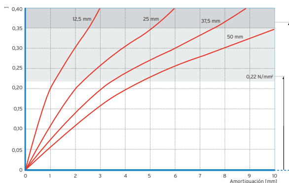
CARGA FLECHA ESTÁTICO
