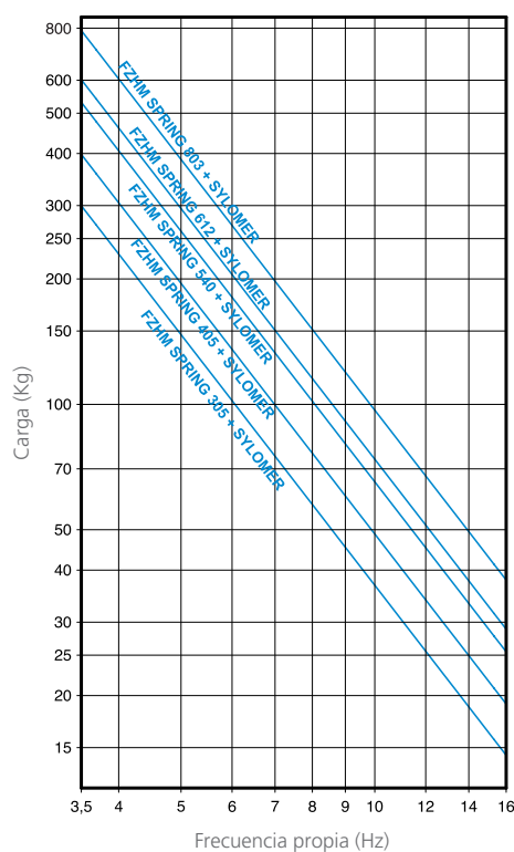
CURVAS DE FRECUENCIA PROPIA FZHM SPRINGS + SYLOMER ®
