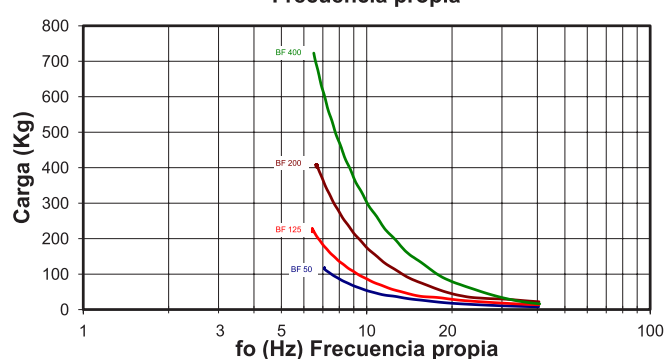
Frecuencia propia
