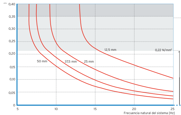
FRECUENCIA PROPIA
