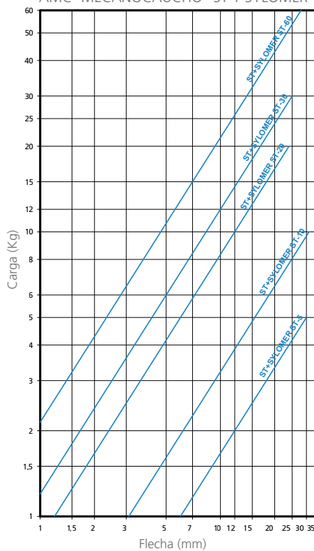
CURVA DE CARGA FLECHA AMC - MECANOCAUCHO® ST + SYLOMER®
