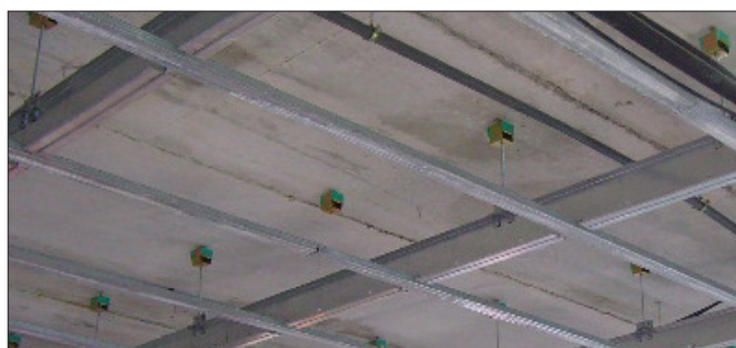
Aplicación de un Akustik 4 + sylomer tipo A
