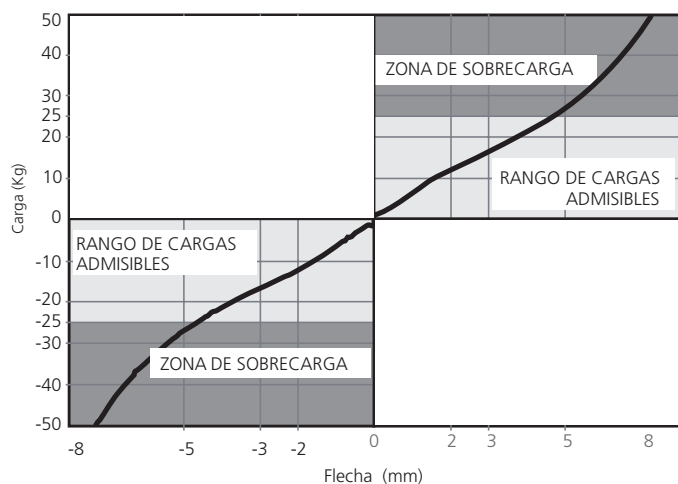
CURVAS DE CARGA FLECHA EP Akustik + Sylomer
