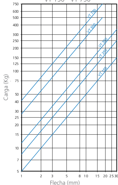
GRÁFICO 1 CARGA FLECHA ESTÁTICO VT 150 - VT 750
