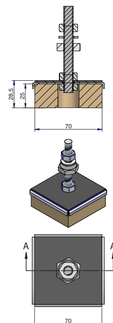
TSR con Kit de Nivelación
