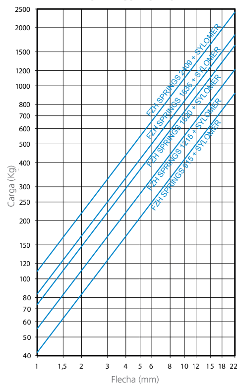
CURVAS DE CARGA - FLECHA FZH SPRINGS + SYLOMER ®
