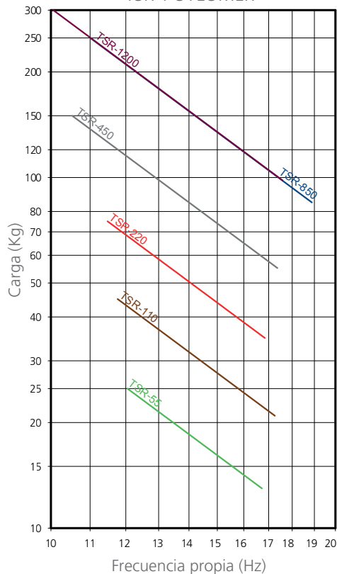
FRECUENCIA PROPIA TSR + SYLOMER ®
