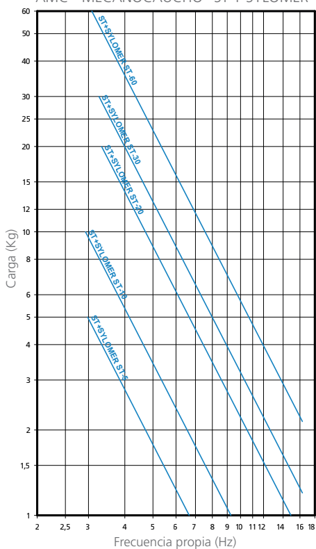
FRECUENCIA PROPIA AMC - MECANOCAUCHO® ST + SYLOMER®
