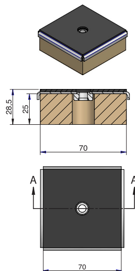
TSR con Kit de Nivelación
