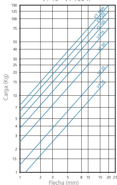
GRÁFICO 1 CARGA FLECHA ESTÁTICO VT 15 - VT 150 R
