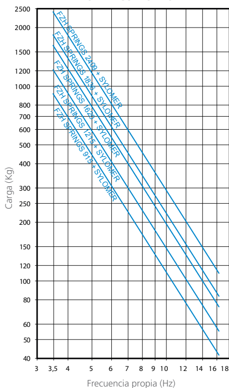
CURVAS DE FRECUENCIA PROPIA FZH SPRINGS + SYLOMER ®
