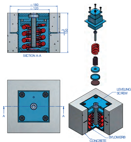
FZH2M + Sylomer ®
