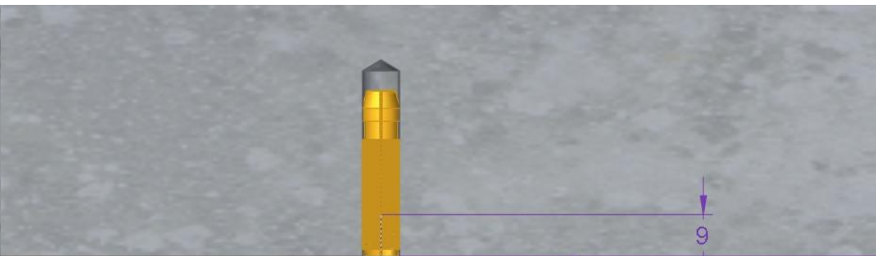
AKUSTIK SUPER T-60 TYP B MINDESTEINSCHRAUBTIEFE IN DÜBEL: 9mm MINDESTABSTAND TRAGDECKE-PROFIL: 86mm
