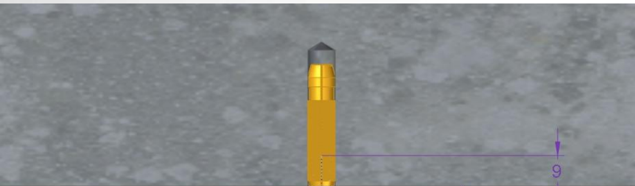
AKUSTIK SUPER T-47 TYP B MINDESTEINSCHRAUBTIEFE IN DÜBEL: 9mm MINDESTABSTAND TRAGDECKE-PROFIL: 77mm
