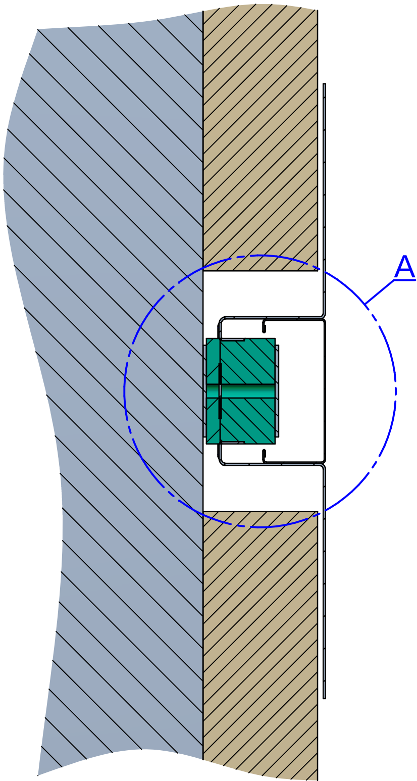
SECTION A-A
