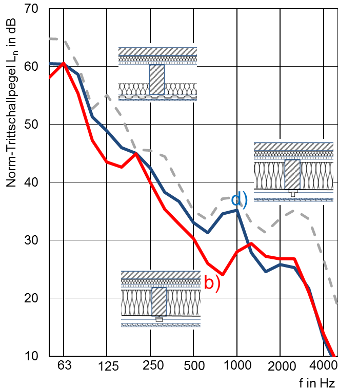
Abbildung 9: Norm-Trittschallpegel der Vergleichsdecke nach Abbildung 5 sowie der optimierten Decken mit den Abhängern b) und d).
