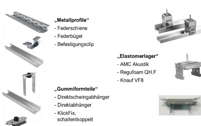
Abbildung 3: Untersuchte Unterdeckenabhängertypen
