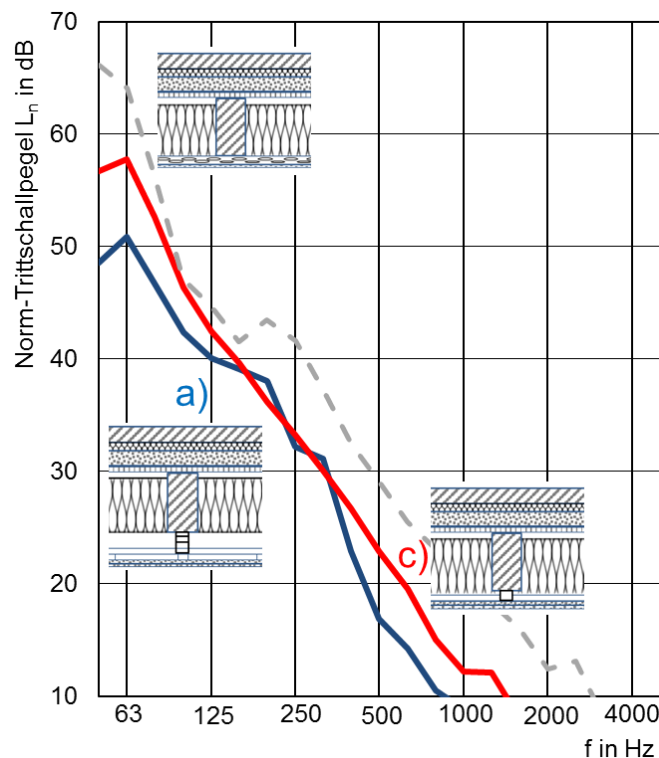
Abbildung 10: Norm-Trittschallpegel der optimierten Aufbauten nach Abbildung 8 mit den Abhängern a) und c) im Vergleich mit einer einlagigen Unterdecke an Federschien.
