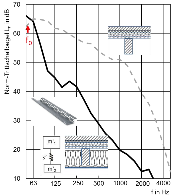
Abbildung 1: Norm-Trittschallpegel einer offenen Holzbalkendecke mit Rohdeckenbeschwerung und schwimmendem Estrich im Vergleich zur gleichen Decke mit abgehängter Unterdecke (Federschiene). Lage der Masse-Feder-Masse Resonanz f_0
