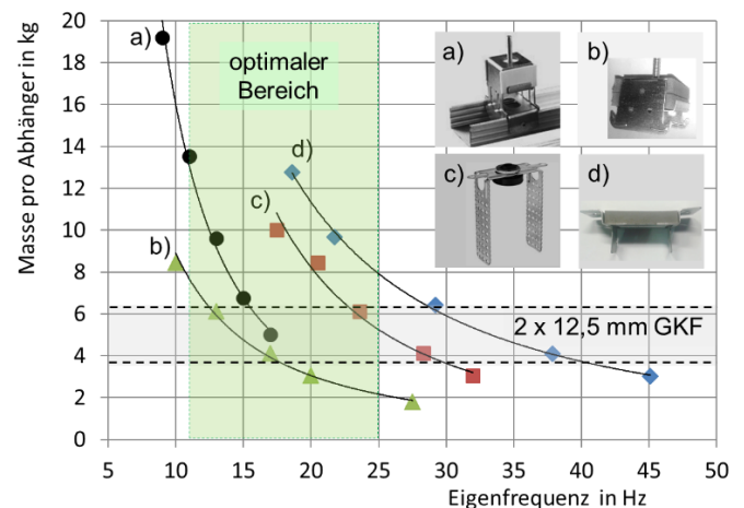
Abbildung 4: Eigenfrequenz unterschiedlicher Unterdeckenabhängertypen in Abhängigkeit der Belastungsmasse in kg/Abhänger. Grün hinterlegt: Optimaler Bereich 12 \text{ Hz} \leq f_{0, \text{Abhänger}} \leq 25 \text{ Hz} . Grau hinterlegt: Typischer Belastungsbereich der Abhänger für eine Unterdeckenbekleidung aus 2 x 12,5 mm GKF
