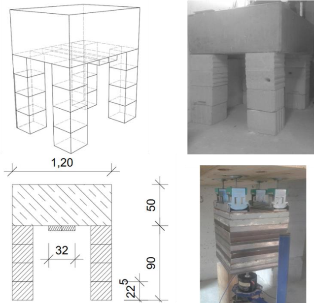
Abbildung 2: Prüfstand zur Ermittlung der Eigenfrequenz von Unterdeckenabhängern. Links: Prinzipskizze und Abmessungen. Rechts unten: Ermittlung der Eigenfrequenz (hier bei maximaler Belastung) durch Anregung mit einem Shaker und Messung der Beschleunigungspegel an 3 Körperschallaufnehmer-Positionen.
